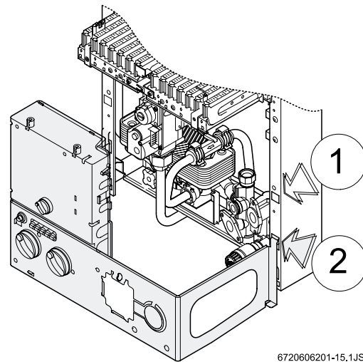
Fig. 20 Poziția service
