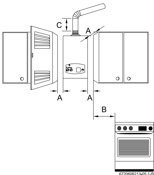
Fig. 6 Distanțe minime
