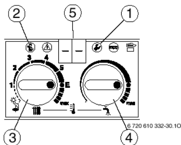
Figura 23 Privire de ansamblu asupra elementelor de comandă
