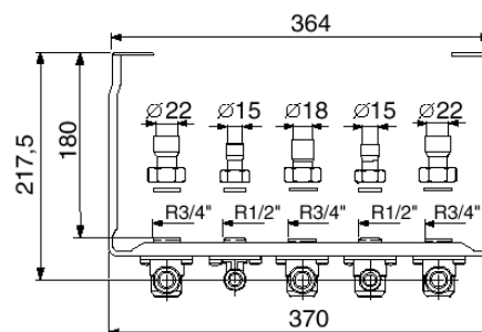
Figura 5 Racordarea conductelor de alimentare
