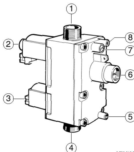
Figura 42 Vana de gaz
