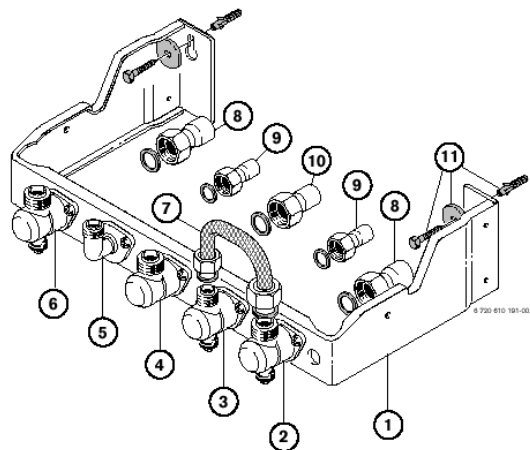
Figura 6 Placa de racorduri
