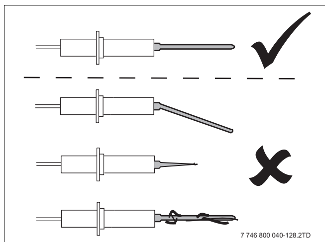
Fig. 110 Verificarea electrodului de ionizare
