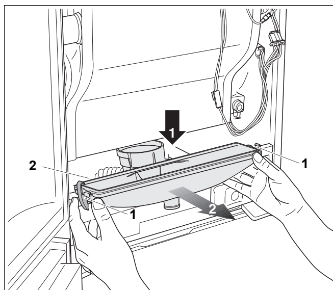
Fig. 115 Scoateți vana de condensat
