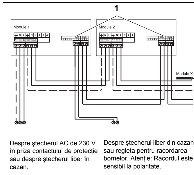
Fig. 49 Racordați mai multe module
