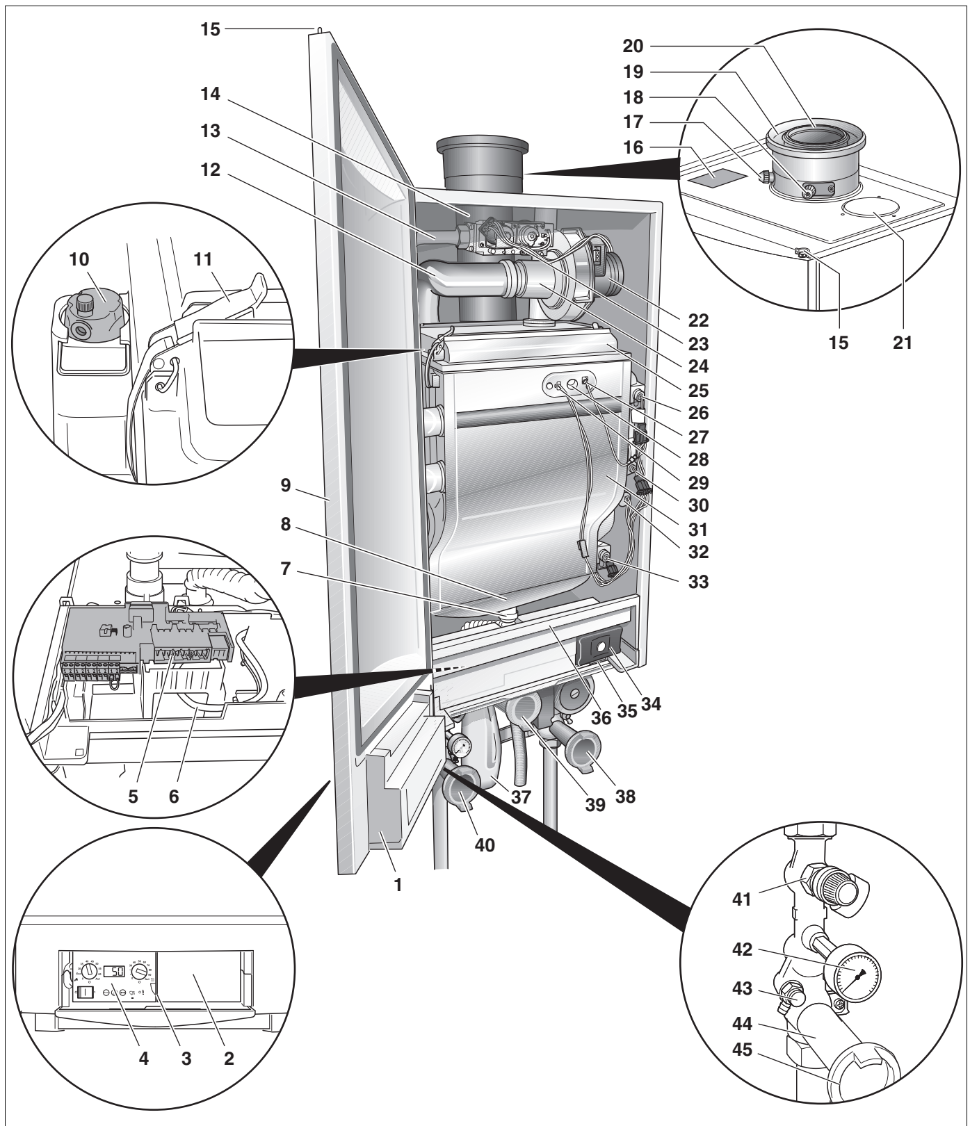
Fig. 1 Logamax plus GB162-65/80/100 cu grup de racord
