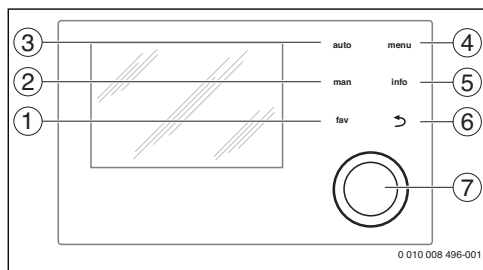
Fig. 1 Elemente de comandă
